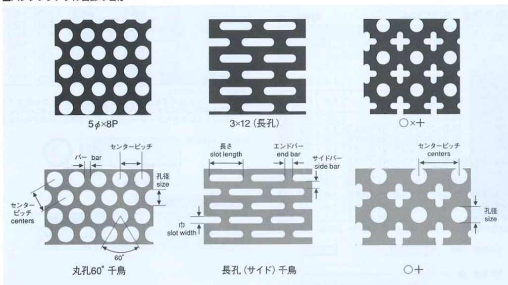
■パンチングメタル各部の名称
