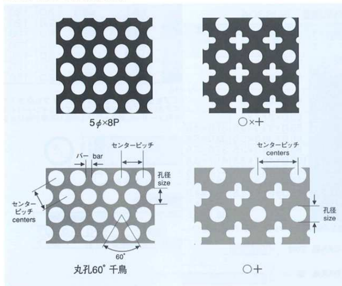
■パンチングメタル各部の名称
